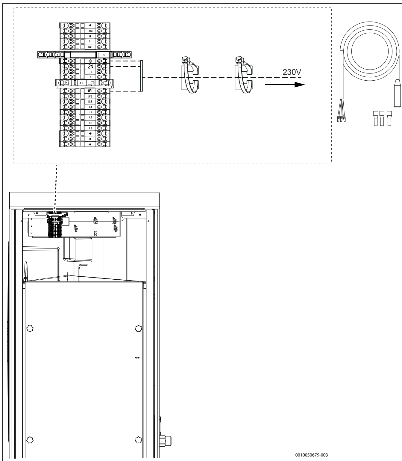
Fig. 39 Varmekabeltilslutning (tilbehør)
