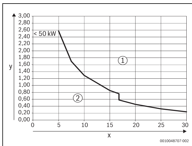
Fig. 19 Varmeproducenter < 50 kW-100 kW
