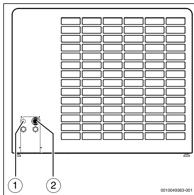
Fig. 36 Kabelforskruninger
