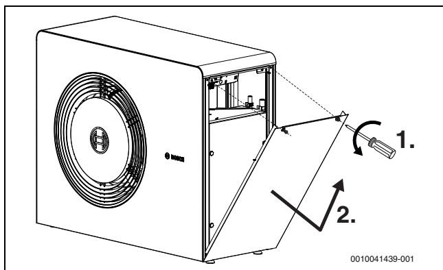
Fig. 31 Sidedæksel
