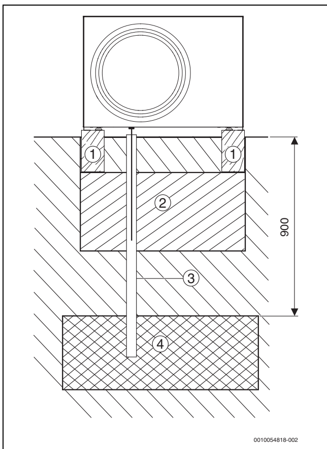
Fig. 28 Kondensatudløb i grusfileret (dimensioner i mm)
