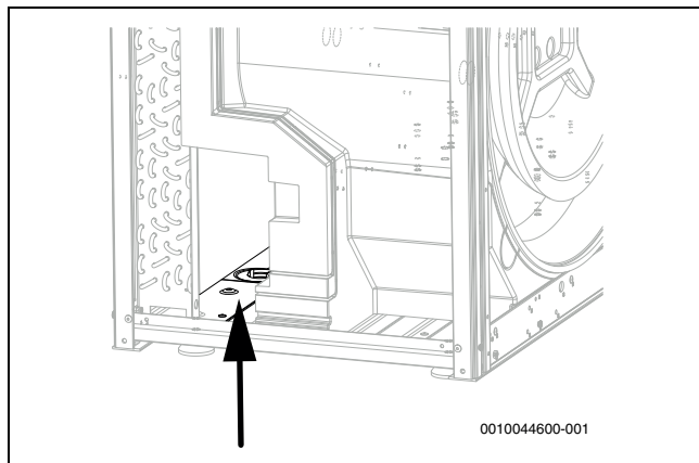
Fig. 42 Rengør drypbakken
