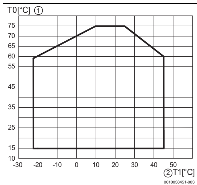
Fig. 44 Varmepumpe i varmedrift uden varmelegeme
