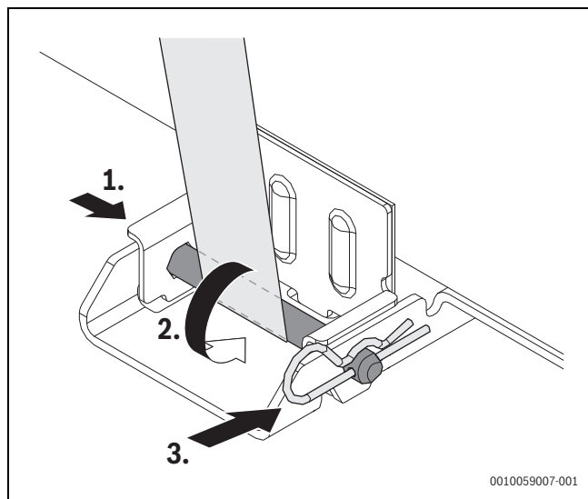
Fig. 13 Indsættelse af låsebeslag, stift og rem
