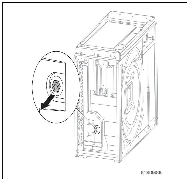
Fig. 40 Skru ud
