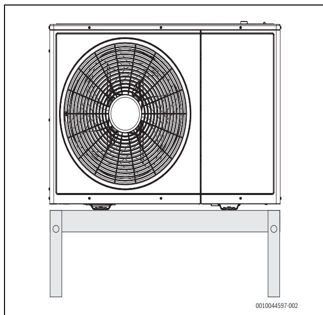
Fig. 21 Varmepumpe på gulvfod
