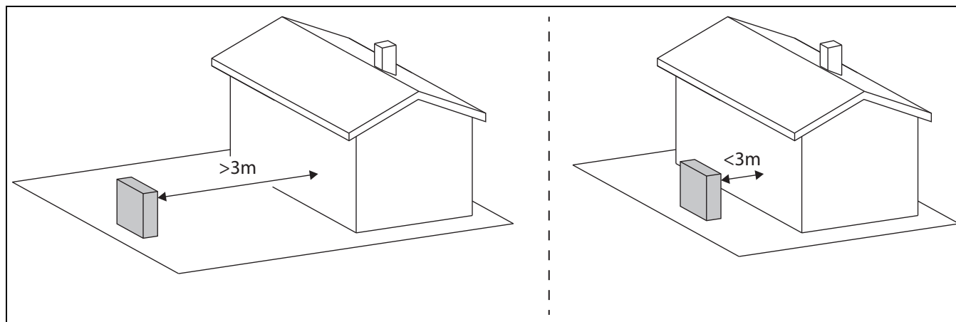
Fig. 43 Afstand til væg
