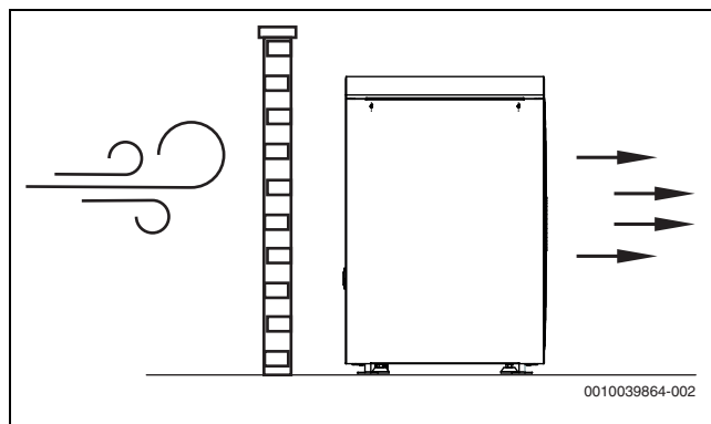
Fig. 17 Fritstående varmepumpe
