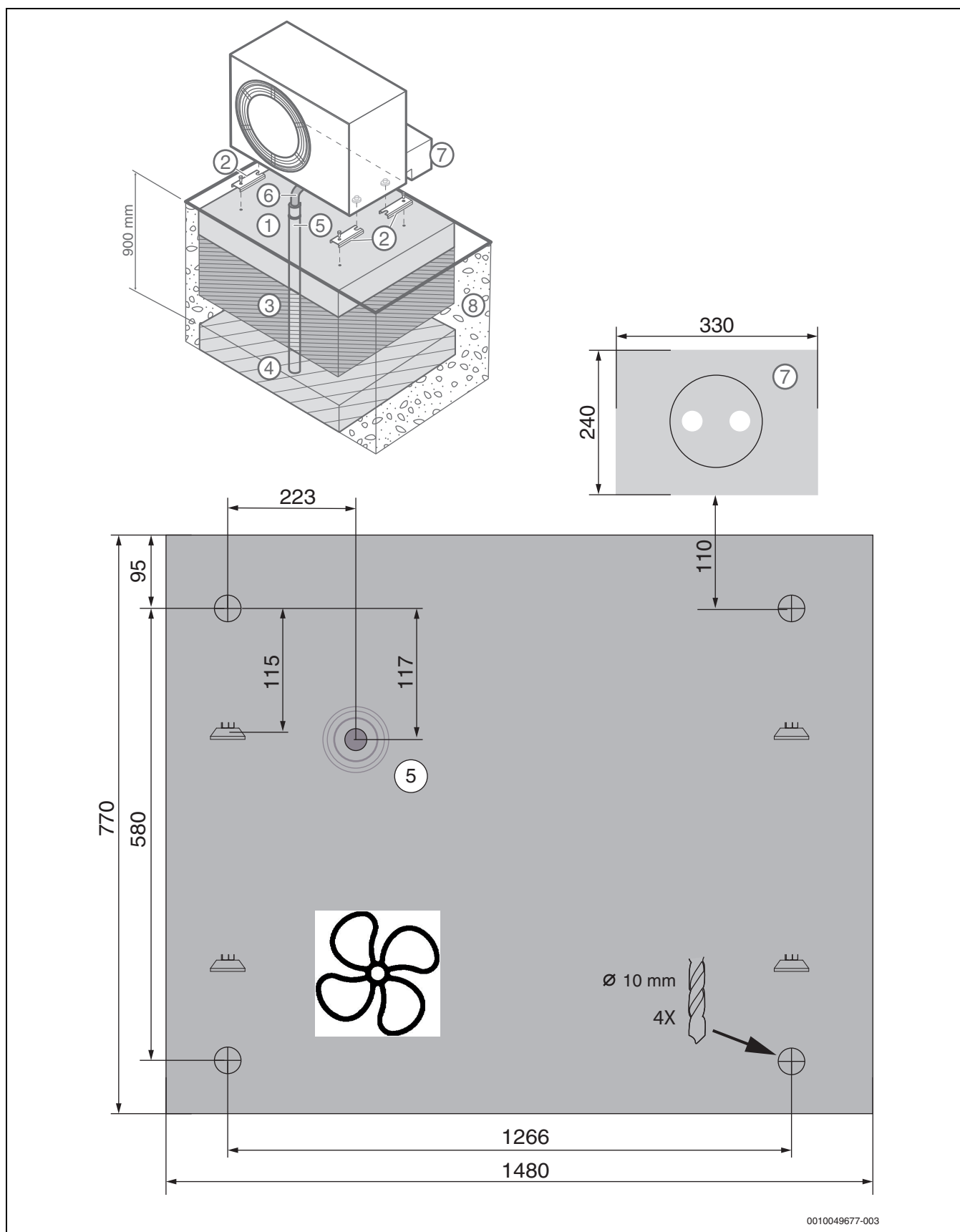
Fig. 25 Fundamentplan, alternativ 2
