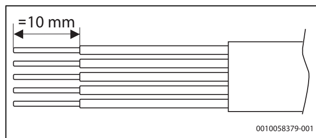
Fig. 37 Afisolering af ledningerne til nettilslutningen
