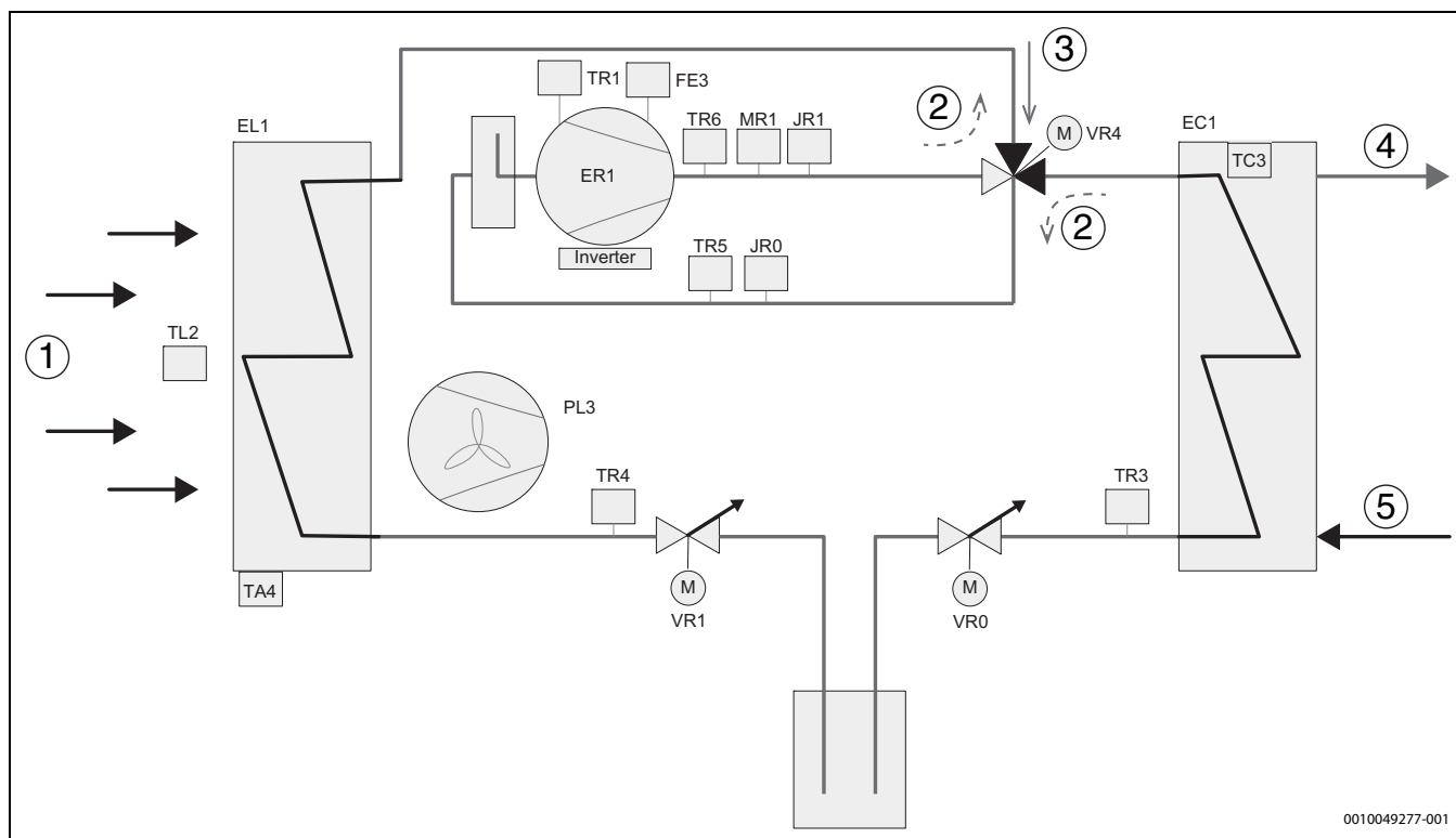
Fig. 46 Kølemiddelkreds
