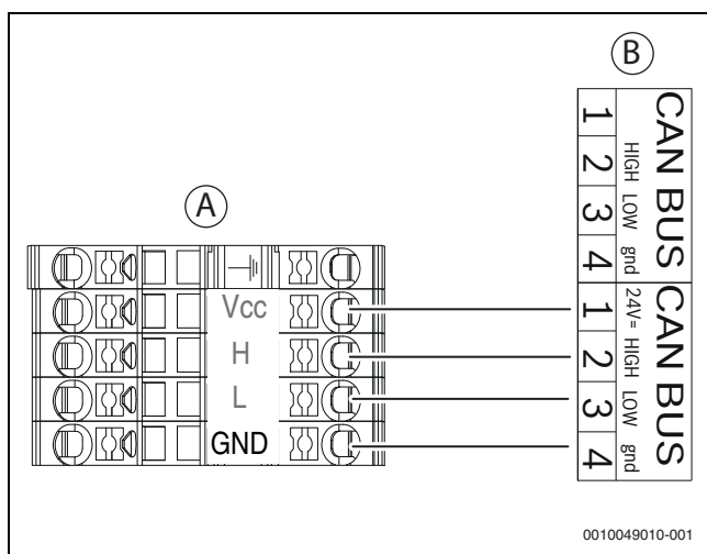
Fig. 34 CAN-BUS til varmepumpe – indendørsenhed
