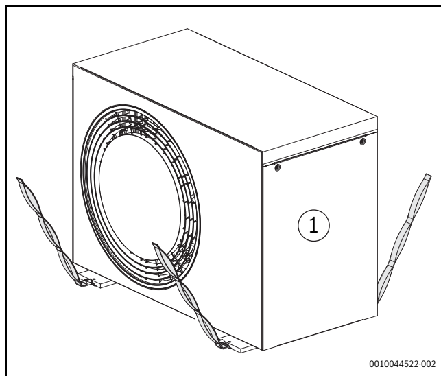
Fig. 11 Anvend remmene, når varmepumpen transporteres uden emballage
