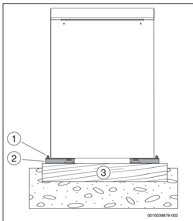
Fig. 20 Fastgørelse af varmepumpen
