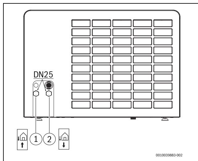
Fig. 30 Tilslutning af varmebærrør; beskrivelsen gælder for alle størrelser
