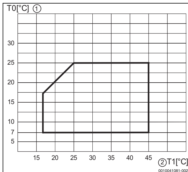
Fig. 45 Varmepumpe i køletilstand
