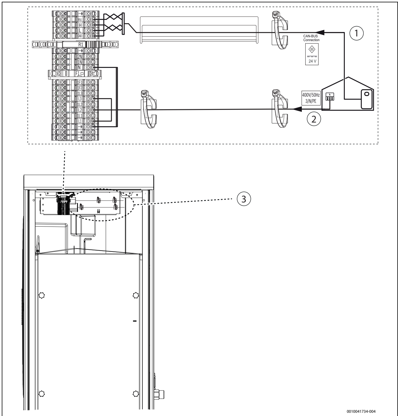
Fig. 38 Klemmer i monteringsområdet
