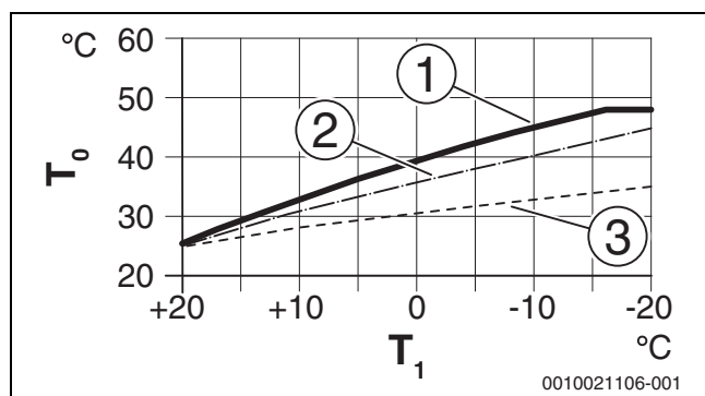
Fig. 2 Indstilling af opvarmningskurve for gulvvarme stigning over vejrkompenserende regulering T_0 og minimale udetemperatur T_{1,min}
