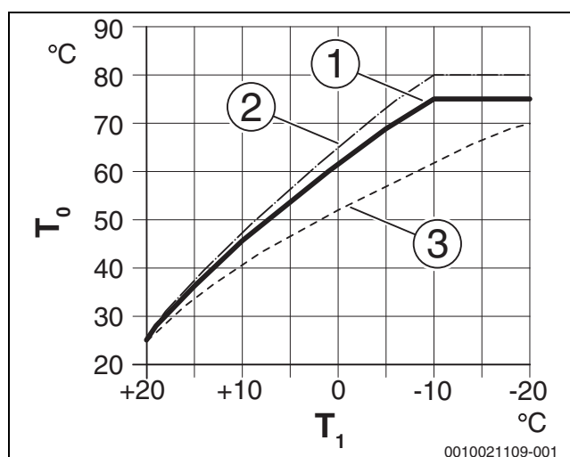
Fig. 4 Indstilling af opvarmningskurven for radiator Stigning over dimensioneringstemperatur T_0 og minimal udetemperatur T_{1,min}
