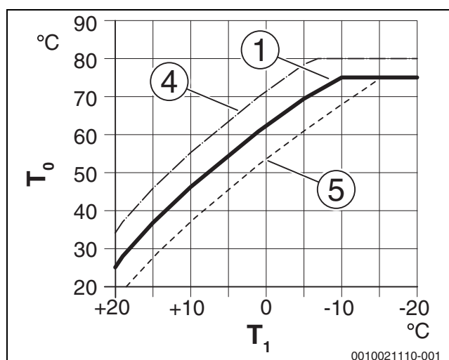
Fig. 5 Indstilling af opvarmningskurve for radiatorer Parallelforskydning over Rumtemperatur-offset eller ønsket rumtemperatur
