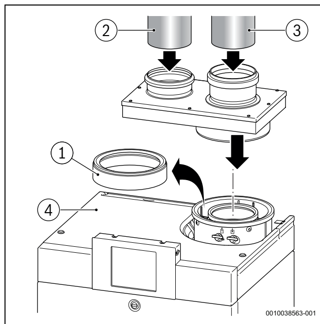
Fig. 2 Monter røggasfløvsadapteren Ø 110-110
